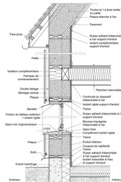
Fig. 4.34. Exemple de coupe verticale d'une paroi avec ossature single-décalée vers l'extérieur
